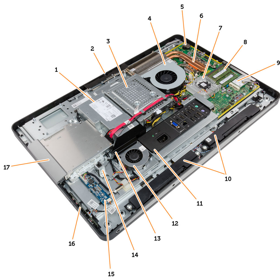
图 1: 内部视图
